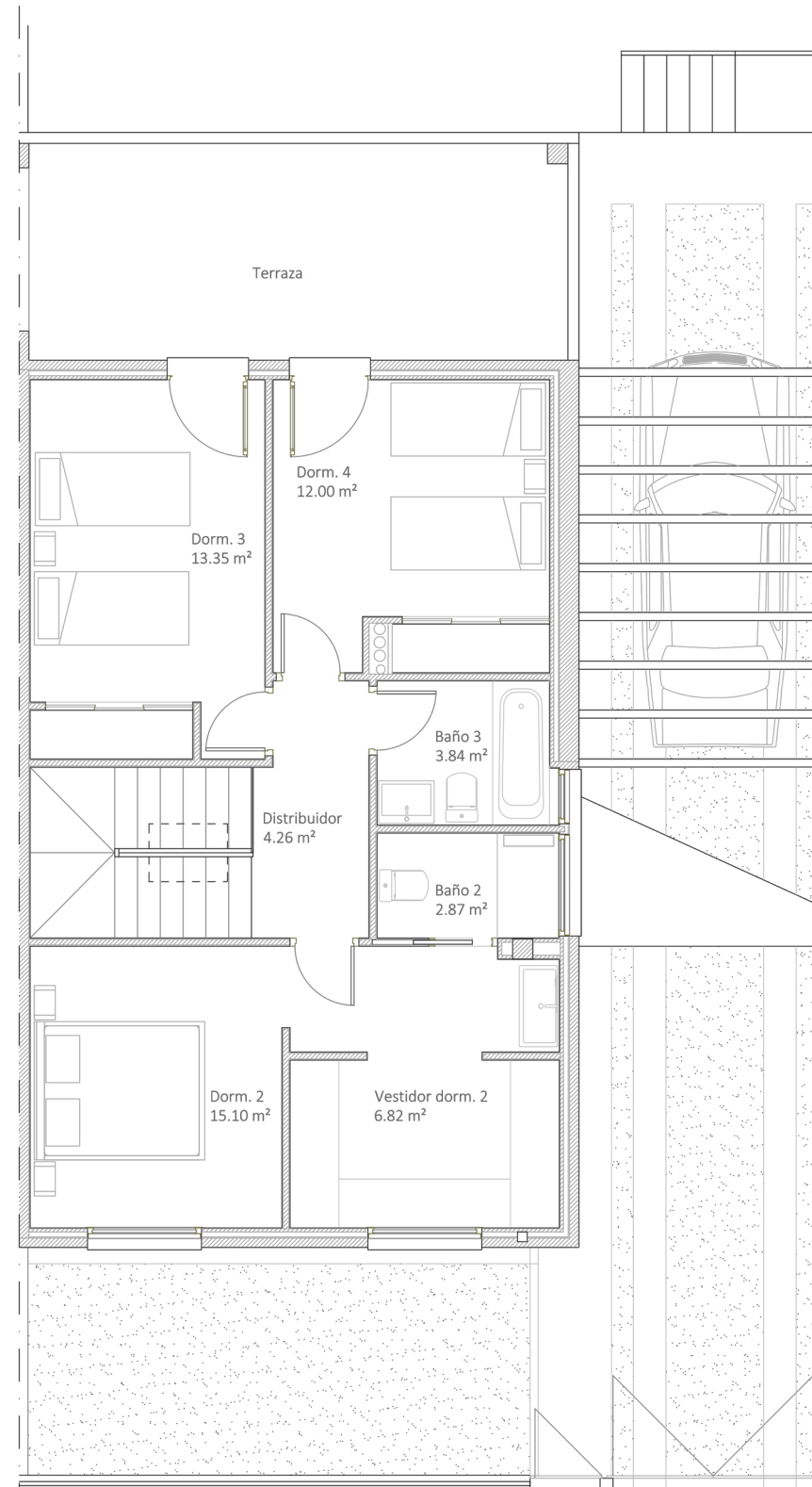
PLANTA PRIMERA
